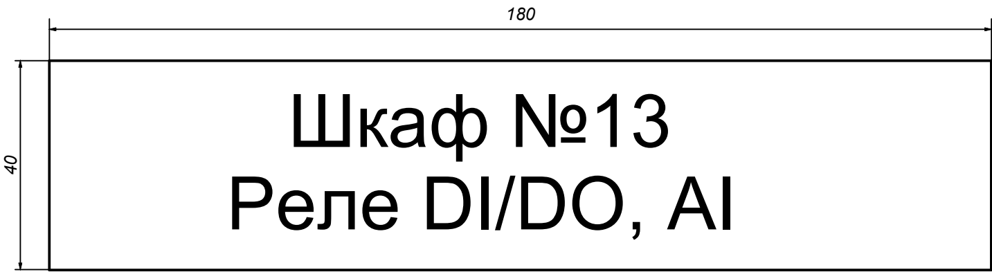
Маркировочный шильдик. Лицевая сторона (1:2)
